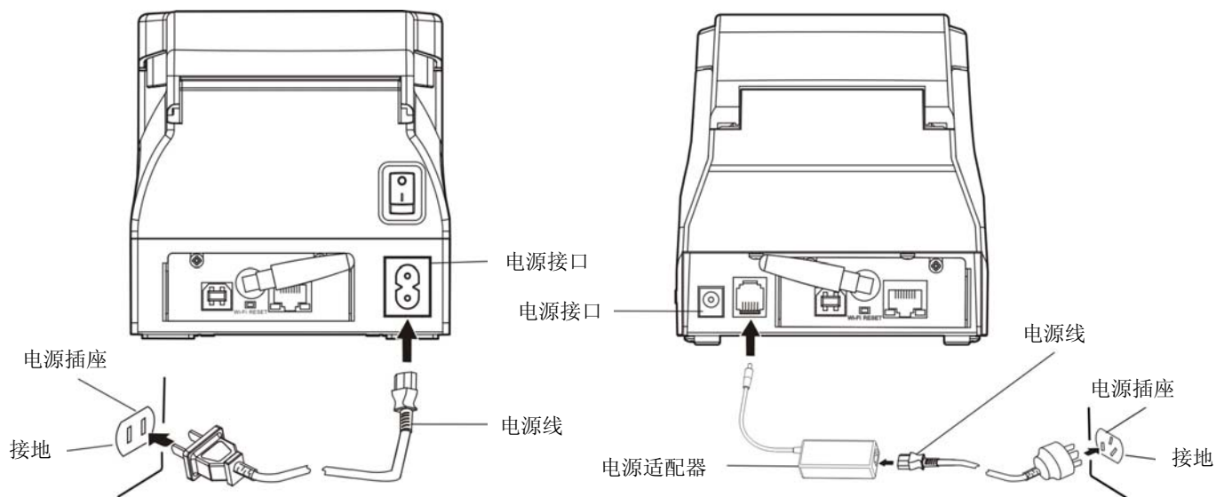
图 2-6 连接电源
